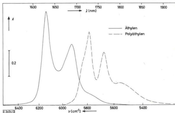
Abb. 3 NIR-Absorptionsbanden von reinem C_2H_4 der Dichte 0,5 \text{ g/cm}^3 und reinem geschmolzenem Polyäthylen im Bereich des ersten Obertons der C-H-Valenzgrundschwingungen
