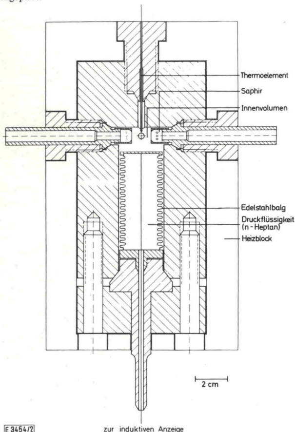
Abb. 2 Optische Hochdruck-Meßzelle
